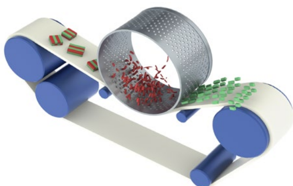
Diagram van het scheidingsproces
